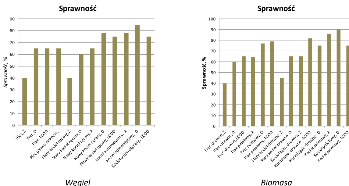
Rys. 19. Sprawność spalania węgla i drewna w różnych urządzeniach grzewczych
