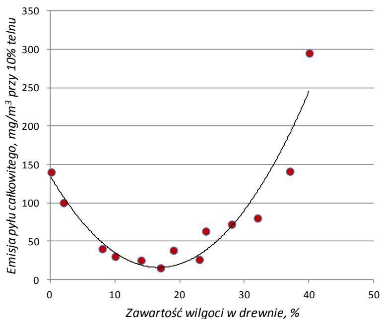
Rys. 28. Wpływ zawartości wilgoci w drewnie na emisję pyłu
