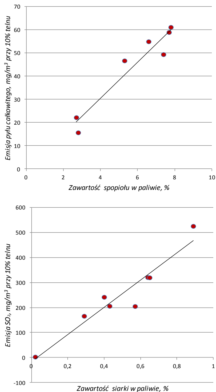
Rys. 27. Wpływa zawartości popiołu i siarki w węglu spalany w kotle z automatycznym załadunkiem paliwa na emisję pyłu oraz SO 2 (mg/m 3 przy 10% O 2 w spalinach)
