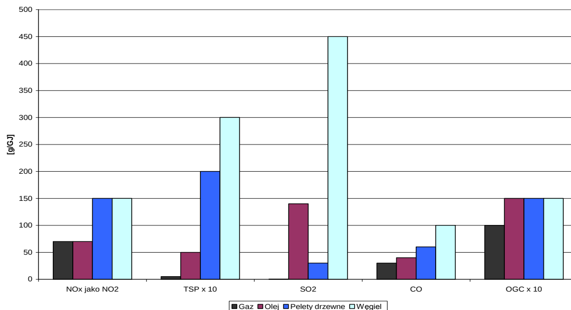
Rys. 16. Porównanie wskaźników emisji NMLZO (OGC), NOx ze spalania paliw stałych – węgla i pelet drzewnych w instalacjach spełniających wymagania BAT (zautomatyzowane kotły małej mocy) oraz gazu i oleju opałowego [g/GJ].
