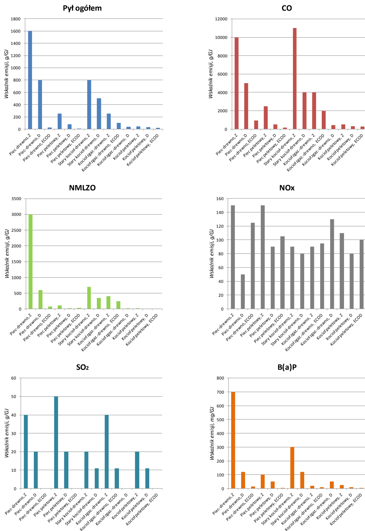
Rys. 18. Emisja zanieczyszczeń ze spalania drewna i pellet w różnych urządzeniach grzewczych Z – stara technika, D- nowa technika, ECOD – wymogi dyrektywy ErP
