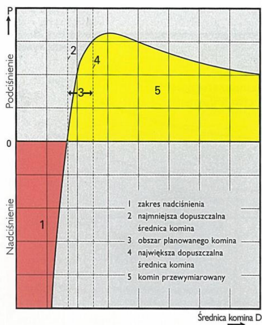
Rys. 32. Doboru rozmiaru komina dla warunków panujących w przewodzie kominowym, z ciągiem naturalnym.
