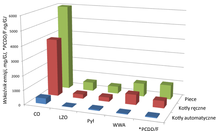
Rys. 7. Wpływ techniki spalania na emisję zanieczyszczeń
