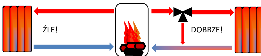
Rys. 36. Zastosowanie zaworu mieszającego
