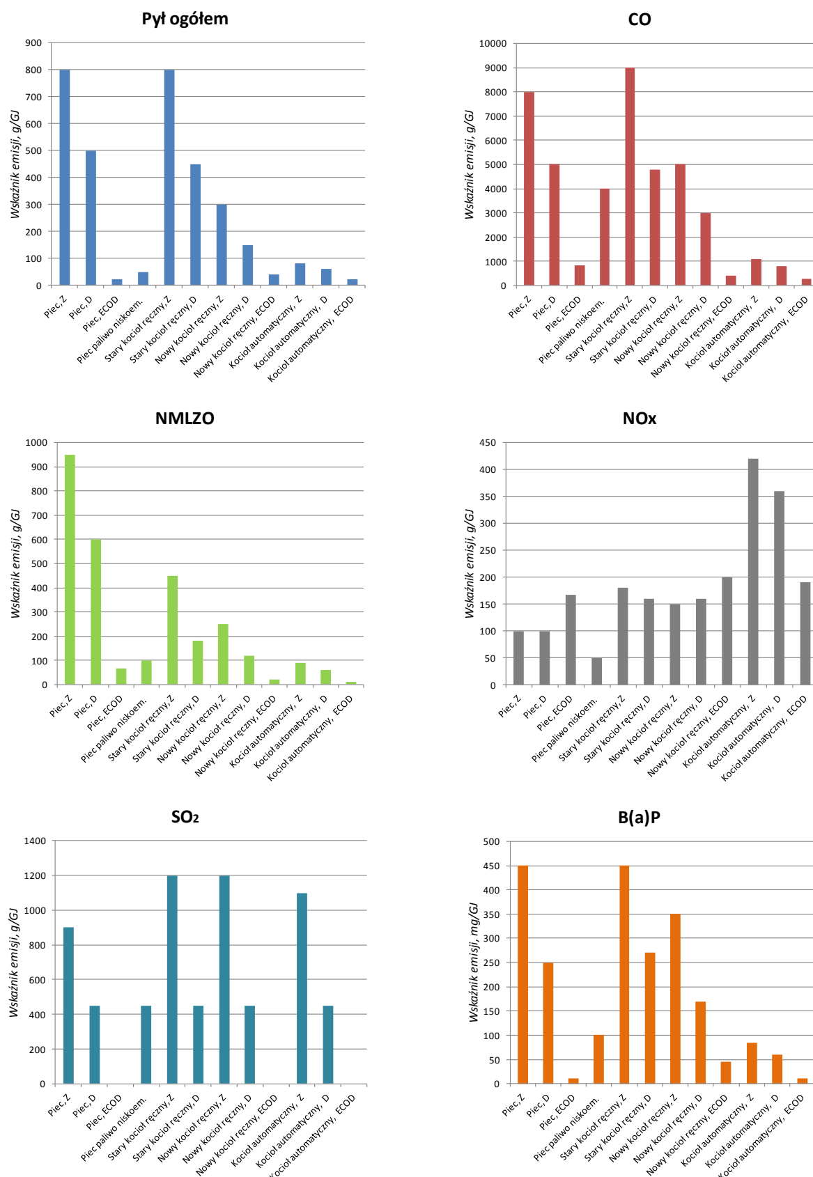
Rys. 17. Emisja zanieczyszczeń ze spalania węgla w różnych urządzeniach grzewczych
