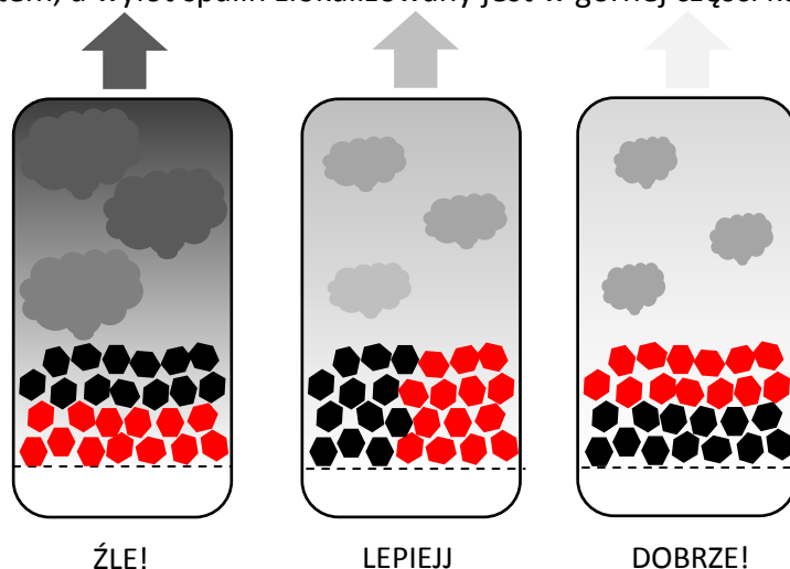
Rys. 35. Sposób spalania dolny vs górny
