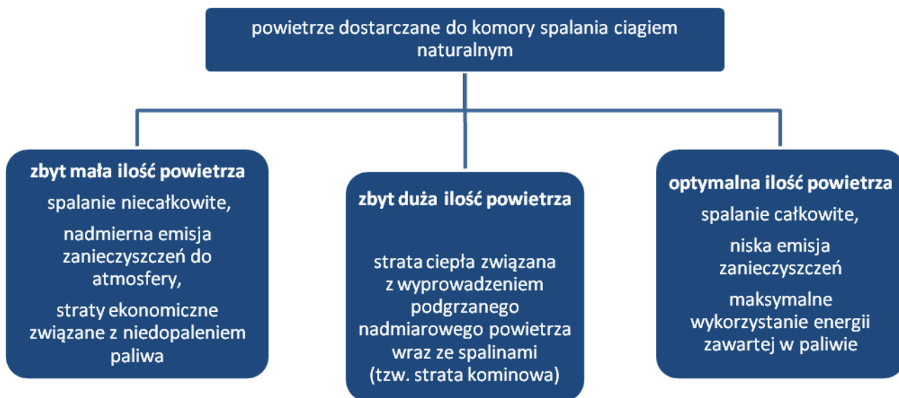
Rys. 33. Wpływ ciągu kominowego na proces spalania
