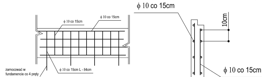
Przekrój przez ścianę
