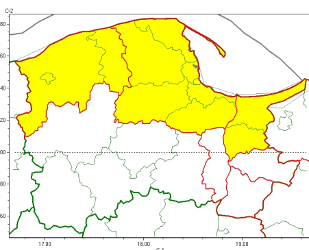
Silny wiatr 2022-12-11 23:43
