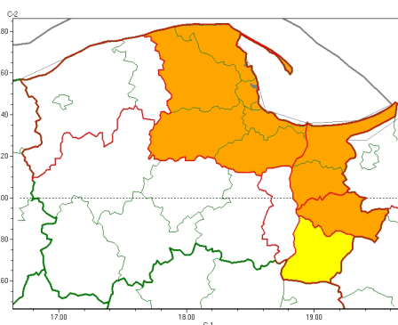
Zawieje/zamiecie śnieżne 2022-12-11 23:43
