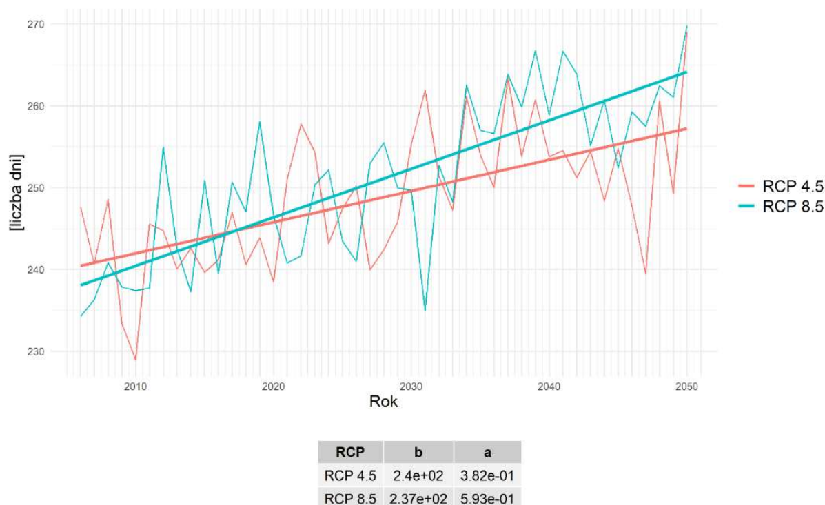
Rys.44. Liczba dni wegetacyjnych ( T_{\text{sr}} > 5^{\circ}\text{C} ), uśredniona dla obszaru Miasta Reda
