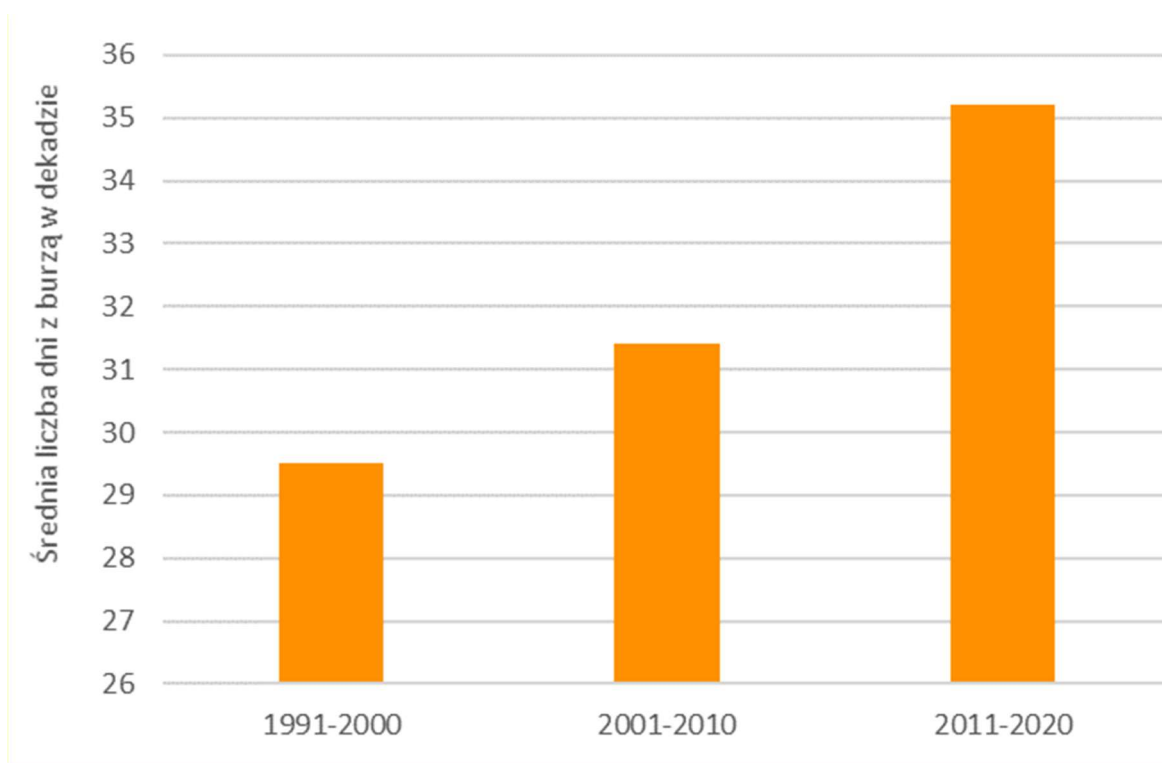
Rys.34. Średnia liczba dni z burzą w wieloleciu, Lębork
