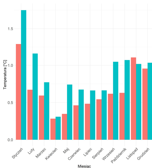
Rys.49. Anomalia średniej miesięcznej temperatury powietrza, uśredniona dla obszaru Miasta Reda; scenariusz RCP 4.5
