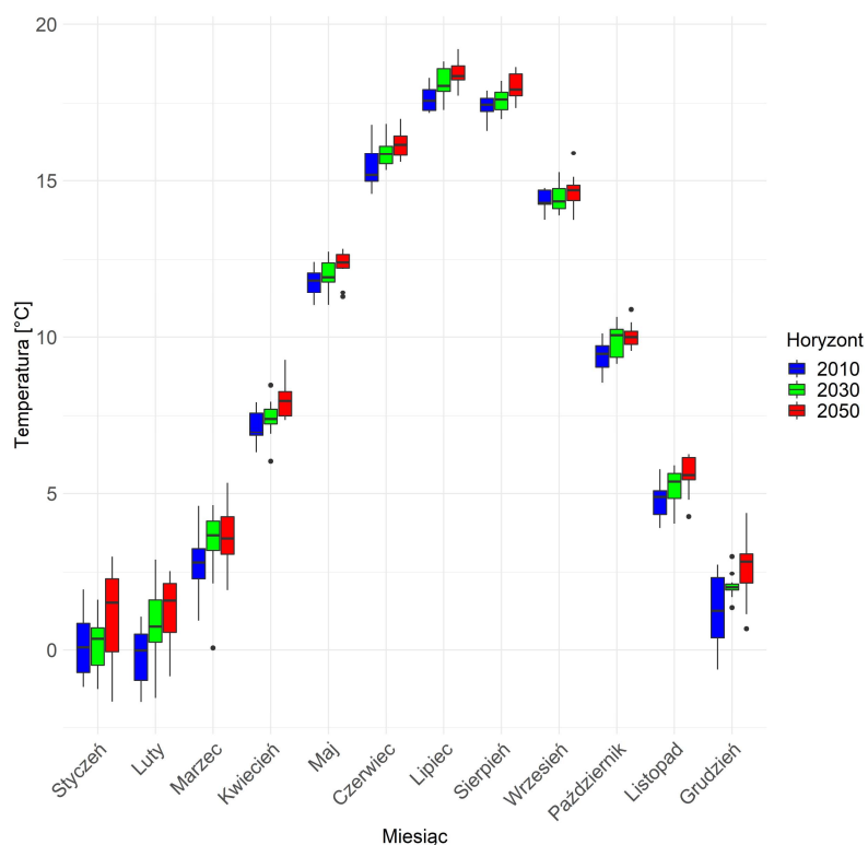
Rys.45. Średnia miesięczna temperatura powietrza, uśredniona dla obszaru Miasta Reda, dla horyzontu roku 2010 – kolor niebieski, dla horyzontu roku 2030 – kolor zielony i dla horyzontu roku 2050 – kolor czerwony; scenariusz RCP 4.5
