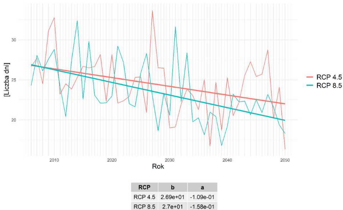
Rys.67. Liczba dni z opadem przy temperaturze od -5°C do 2,5°C, uśredniona dla obszaru Miasta Reda
