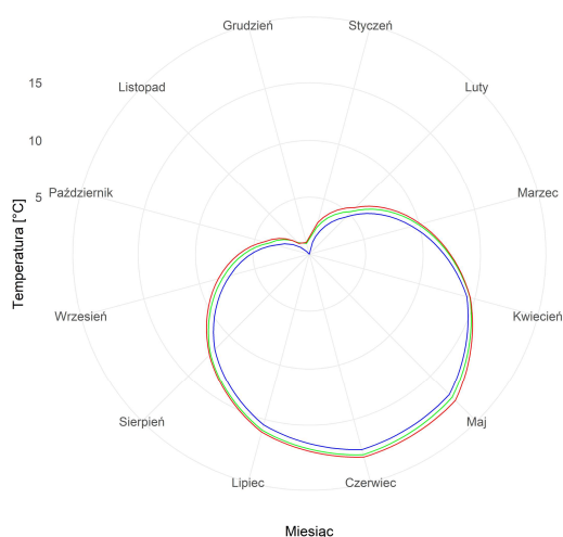
Rys.47. Średnia miesięczna temperatura powietrza, uśredniona dla obszaru Miasta Reda, dla horyzontów 2010, 2030 oraz 2050; scenariusz RCP 4.5
