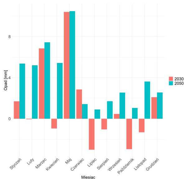
Rys.73. Anomalia sumy miesięcznej opadu, uśredniona dla obszaru Miasta Reda; scenariusz RCP 8.5
