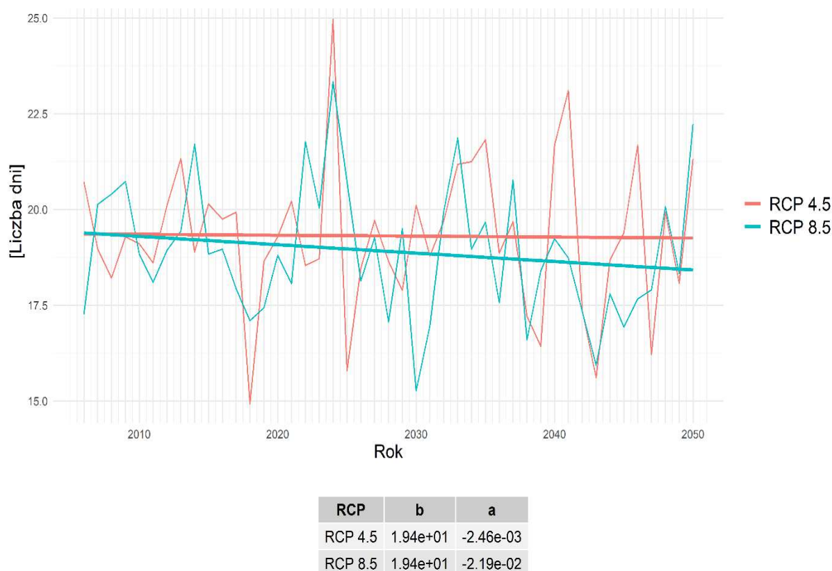
Rys.89. Najdłuższy okres bez opadu, uśredniony dla obszaru Miasta Reda
