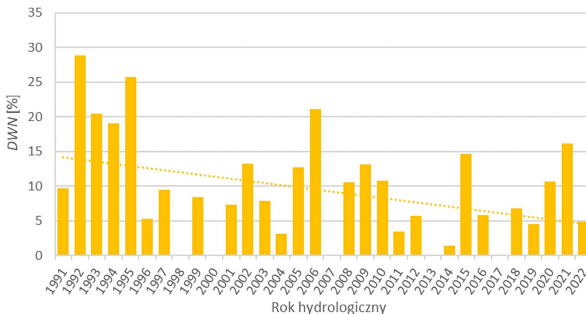
Rys.95. Deficyt względny odpływu niżówkowego w poszczególnych latach hydrologicznych (profil Wejherowo, rz. Reda)
