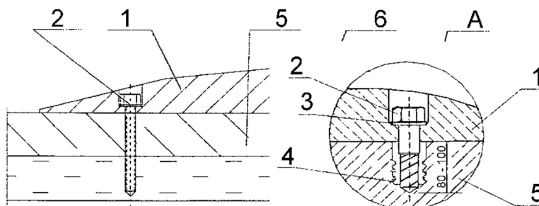
Szczegół A
