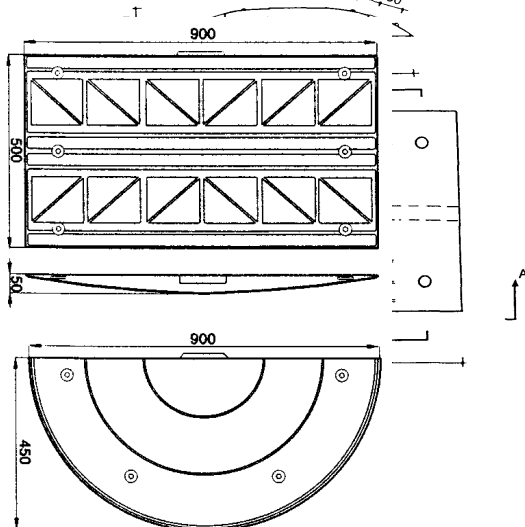
środkowy 500 mm
